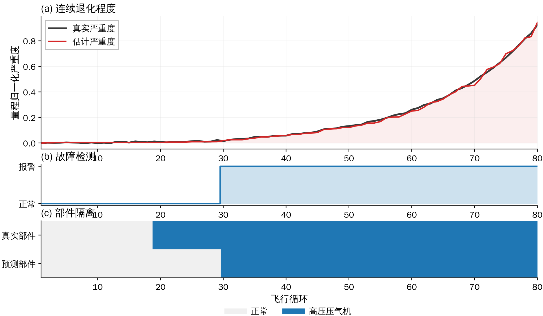
代表发动机从退化出现到部件判定的诊断时间线
