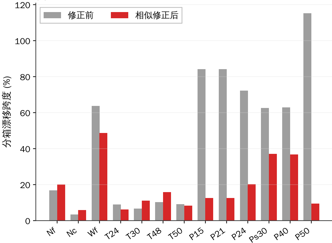
(a) 13 个气路通道的工况漂移
