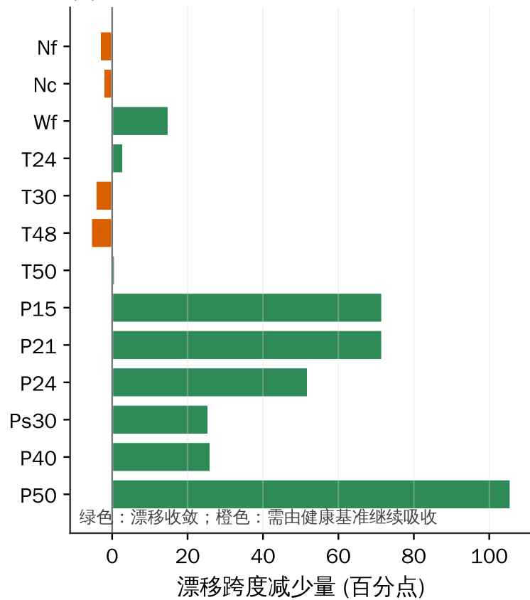
(b) 修正收益及剩余通道偏差
