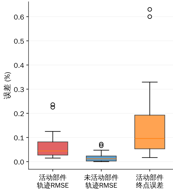
(b) 多口径误差分布
