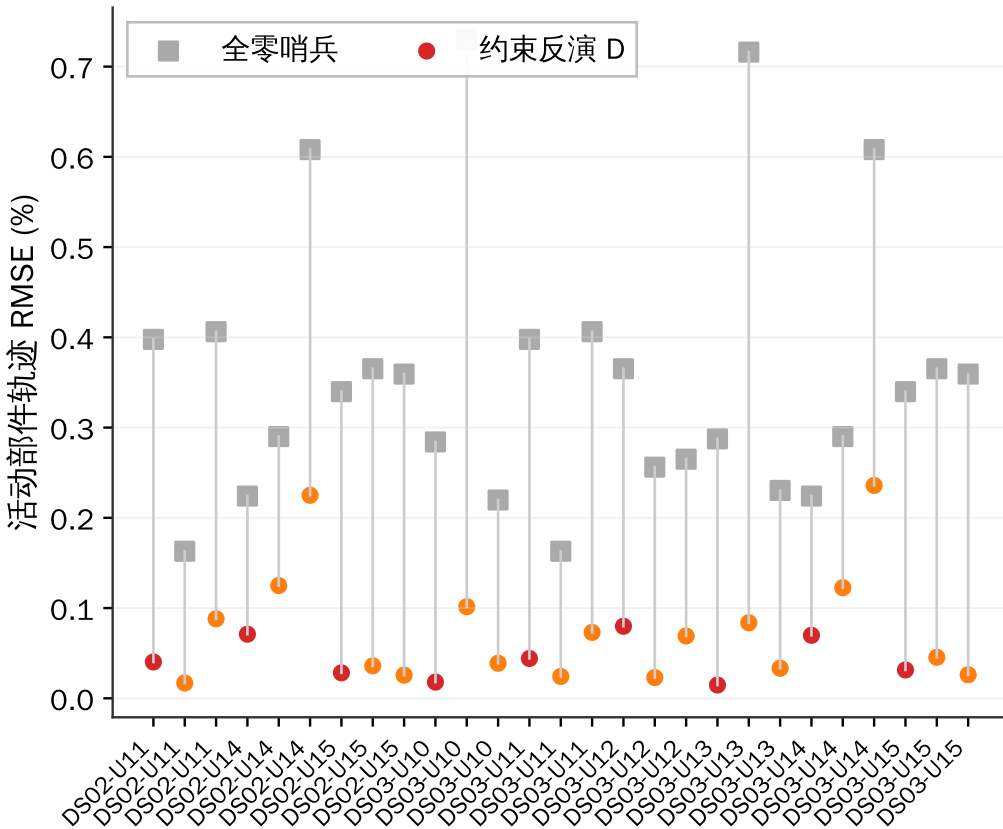
(a) 跨发动机活动部件误差
