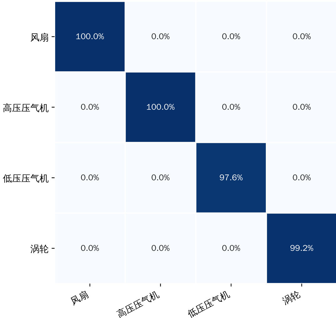
四部件主诊断逐类召回/共现矩阵
