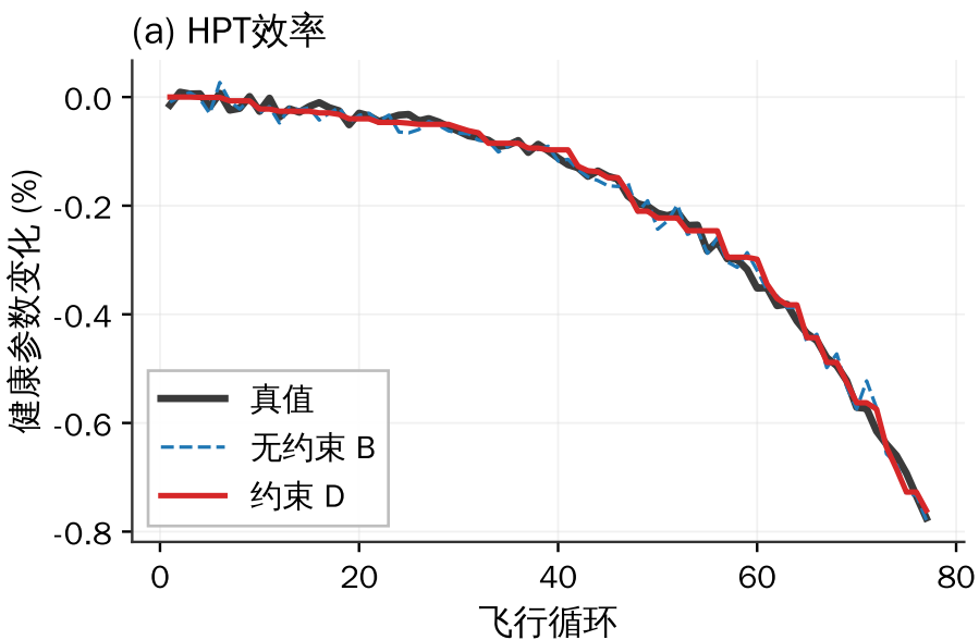
代表发动机连续退化轨迹：相关系数 0.996，RMSE 0.056%
