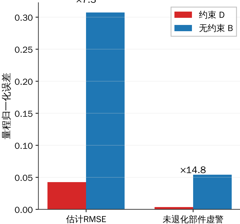
(a) 硬约束的独立价值
