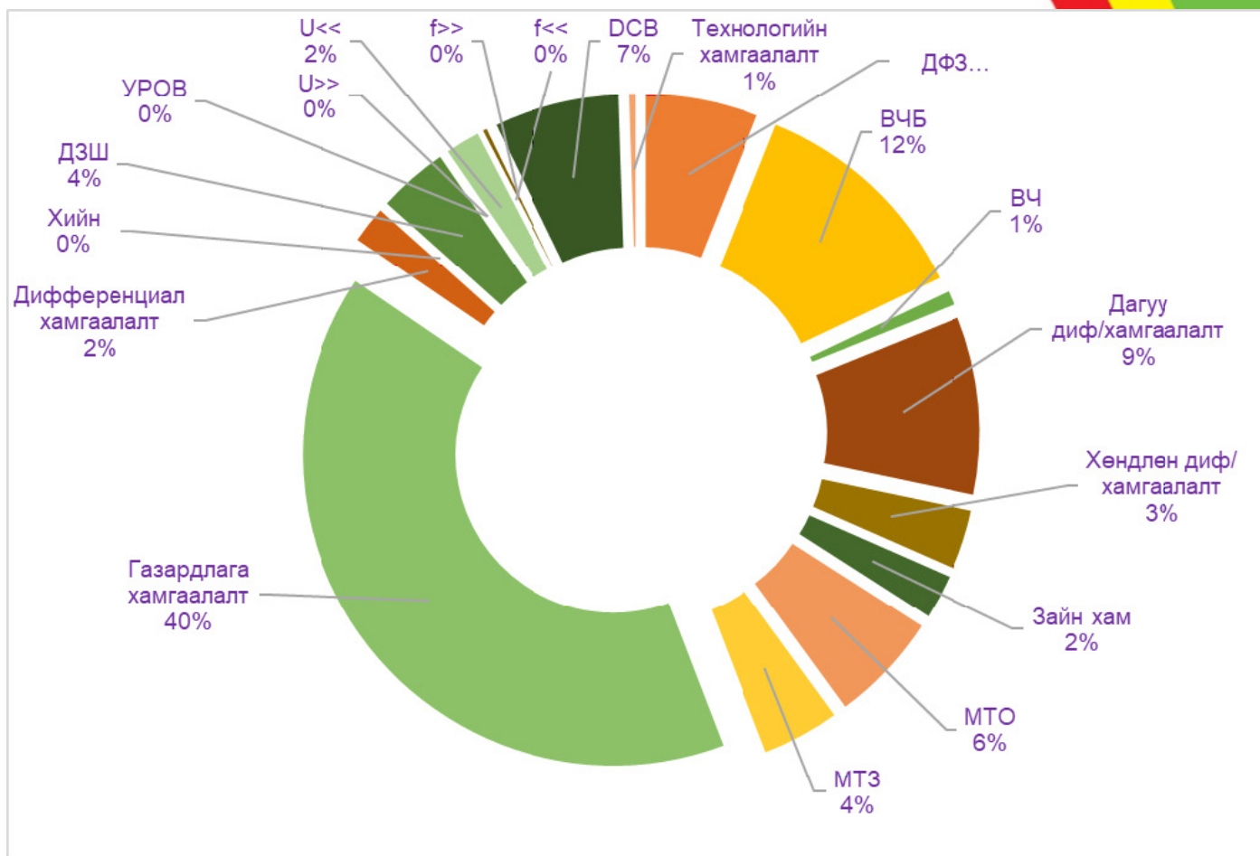
Реле хамгаалалтын ажилгааны төрлөөр
