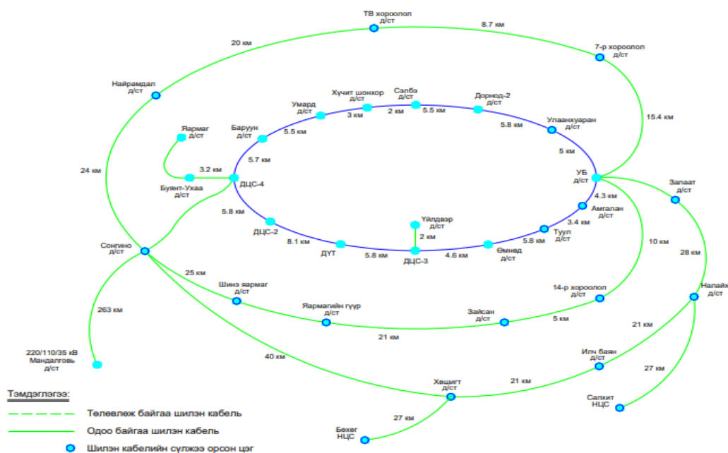
Шилэн кабелийн холболтын бүдүүвч схем
