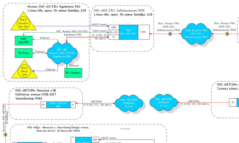
ОХУ-ын БЭХС болон ДҮТ ТӨХХК-ийн хооронд мэдээлэл солилцож байгаа холболтын бүдүүвч схем
