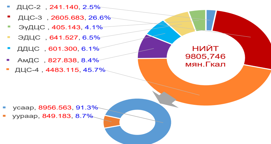
ТБНС-ний 2022 онд түгээсэн ДЭХ
