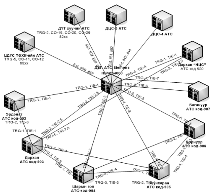
Холбооны системийн АТС-н холболтын зарчмын схем
