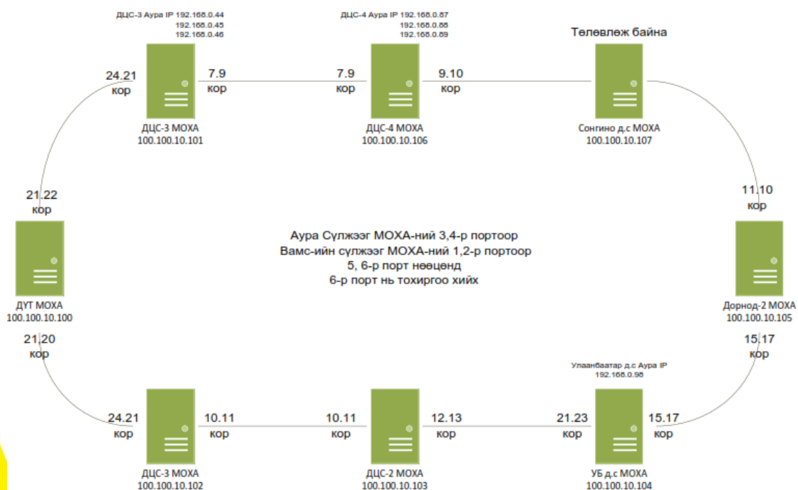
WAMS болон АУРА-н бие даасан сүлжээ үүсгэхээс өмнөх схем
