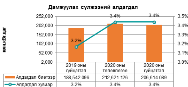
Зураг 4. Сүлжээний алдагдал
