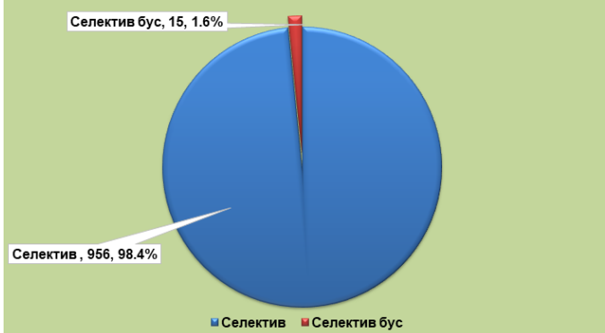
Реле хамгаалалтын ажиллагааны нэгдсэн үзүүлэлт /2021 онд/
