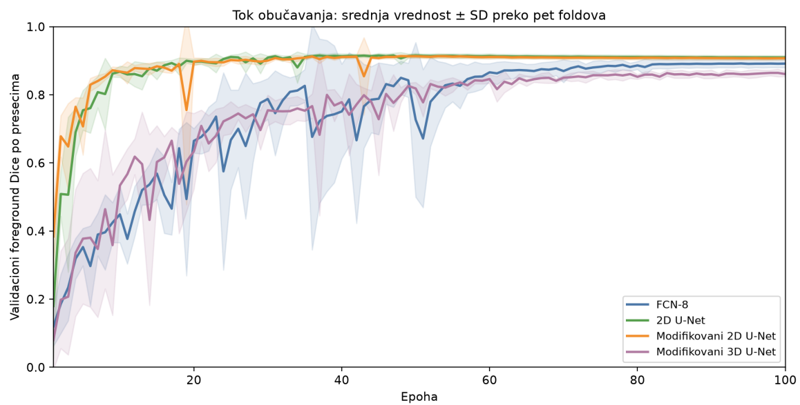
Slika 7: Srednji validacioni foreground Dice po preseccima tokom obuke; osenčeni pojas je SD između foldova.
