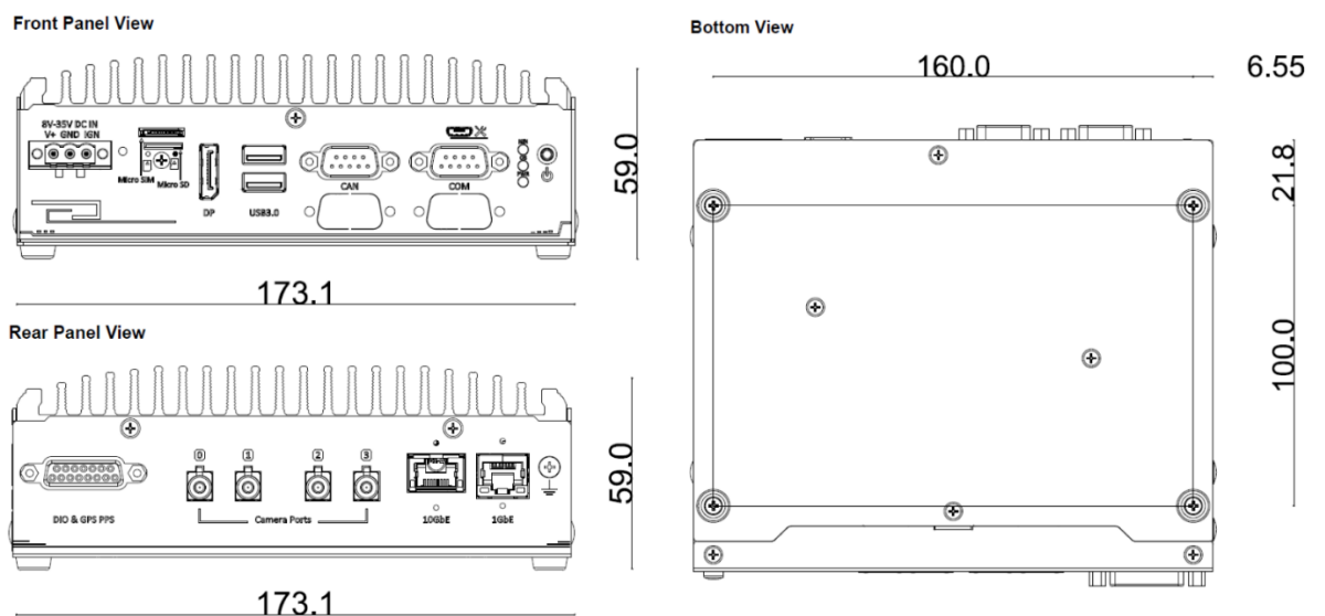
รูปที่ แสดงขนาดของ Neousys NRU-51V (NVIDIA Jetson Xavier NX) ในหน่วยมิลลิเมตร
