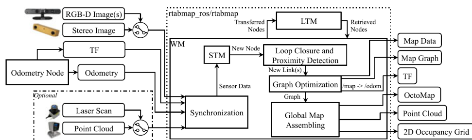
รูปที่ องค์ประกอบหลักในระบบ RTAB-MAP
