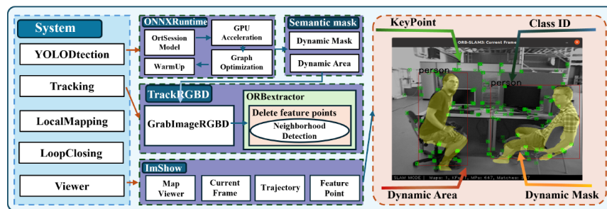
รูปที่ รายละเอียดของเฟรมเวิร์ก Semantic Segmentation ใน RY-SLAM และกระบวนการทำงานแบบ Multi-Threaded
