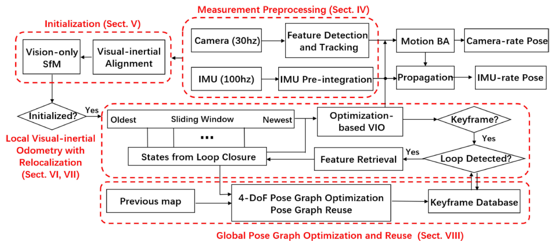
รูปที่ องค์ประกอบหลักในระบบ Monocular VINS
