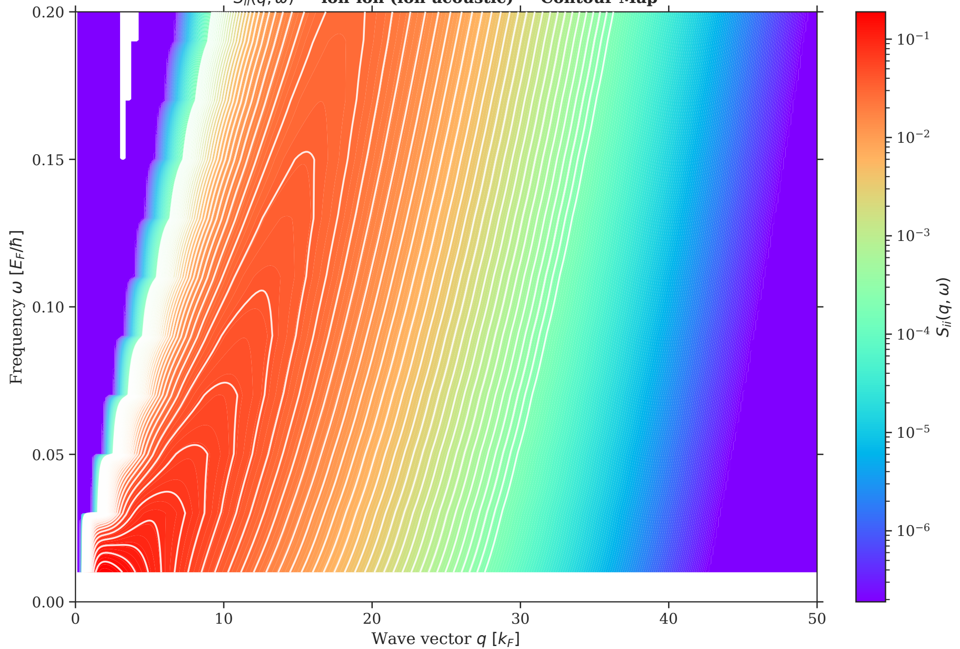
S_{ij}(q, \omega) — ion-ion (ion-acoustic) — Contour Map
