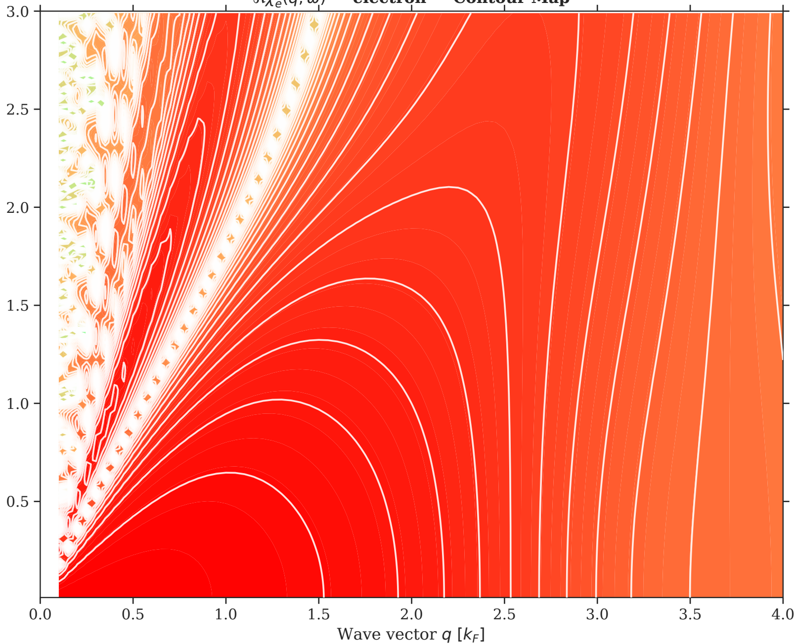
\Re\tilde{\chi}_e^L(\bar{q}, \bar{\omega}) — electron — Contour Map
