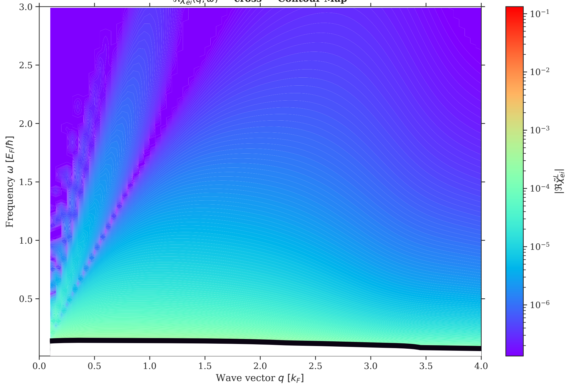
\Re \tilde{\chi}_{ei}^L(\vec{q}, \vec{\omega}) — cross — Contour Map
