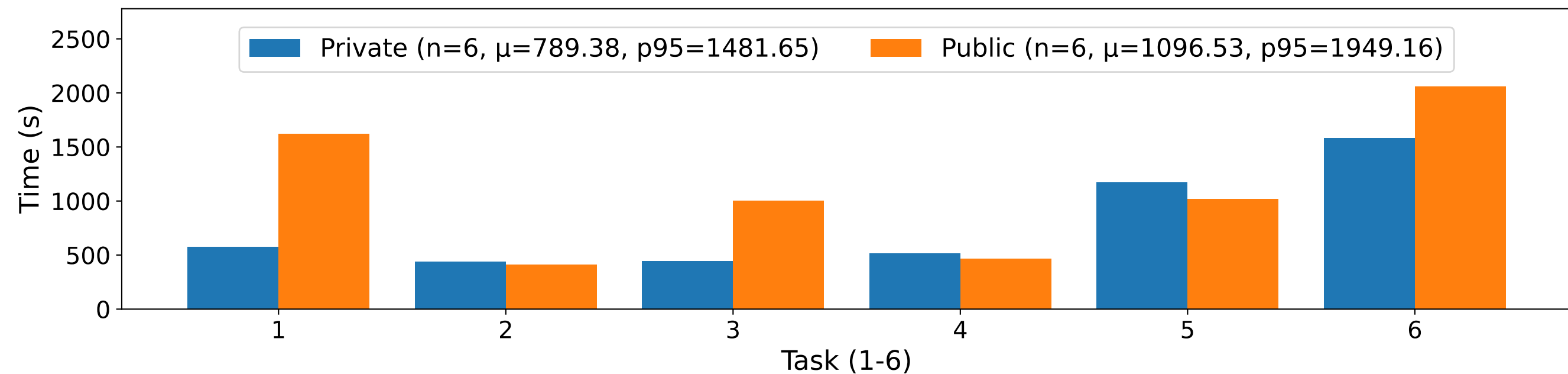
Phi-4-mini*
