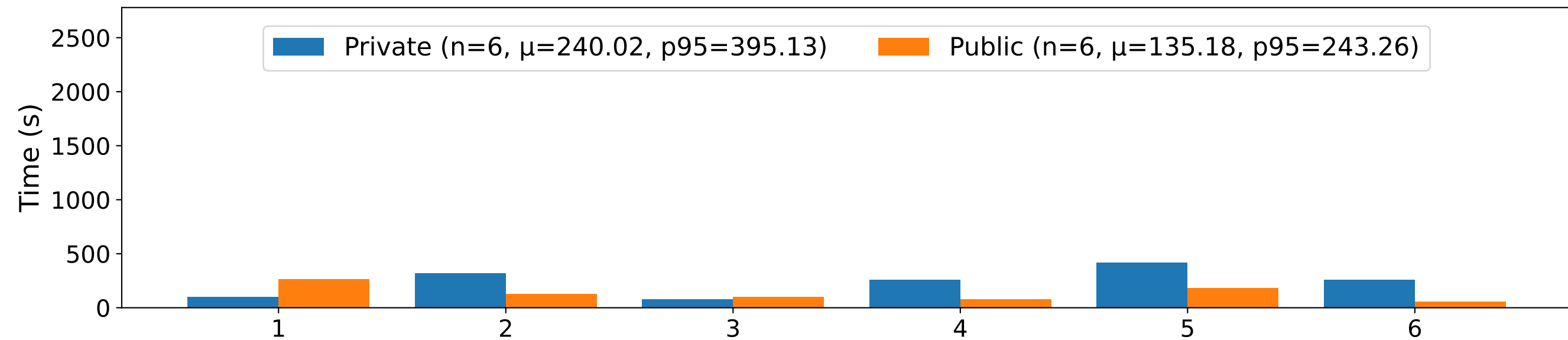
GPT-4o-mini
