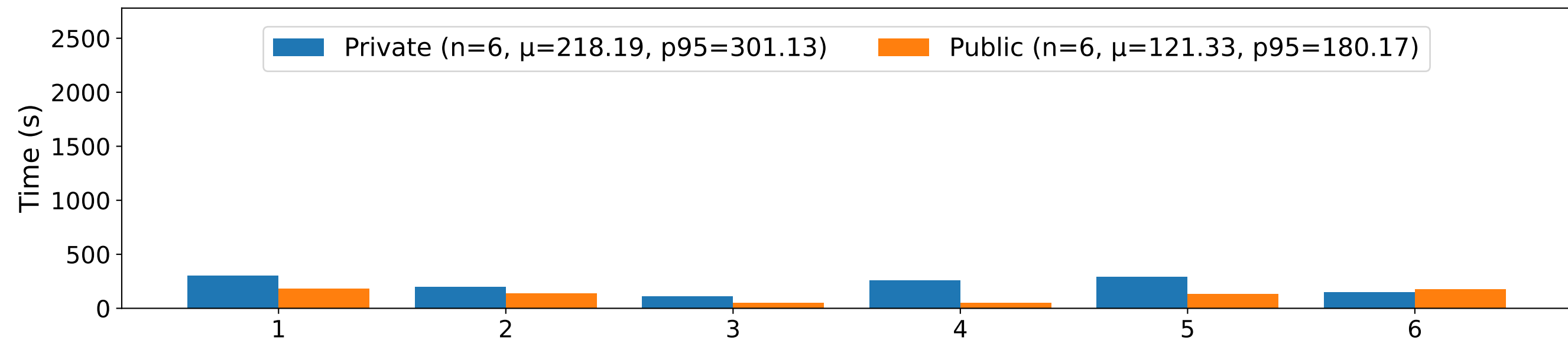
Phi-4-mini*
