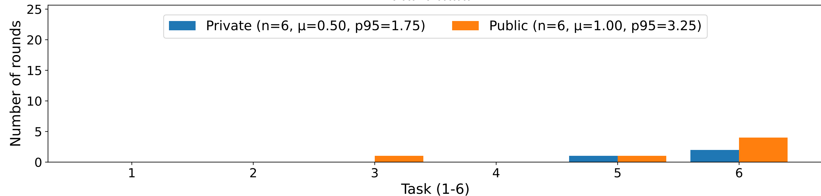
Phi-4-mini*
