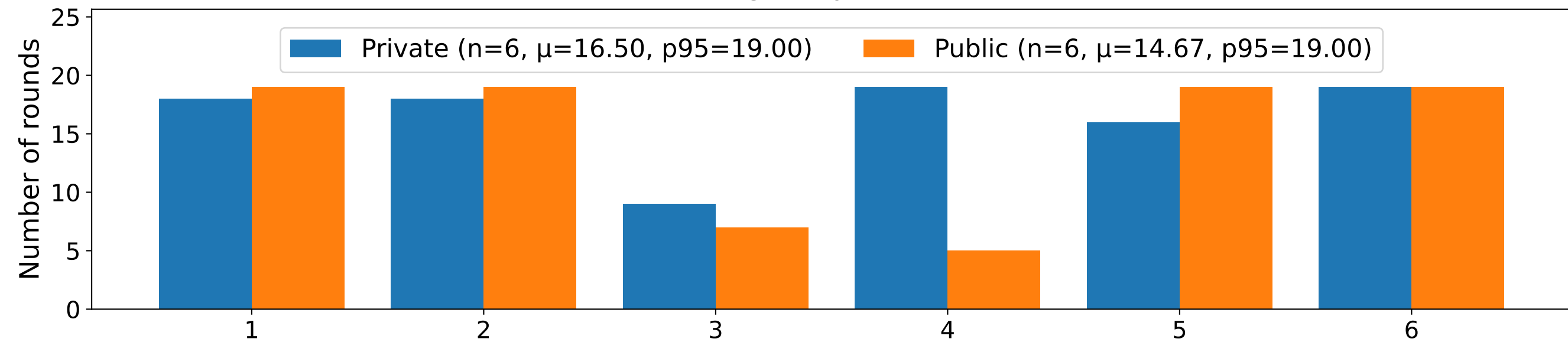
Phi-4-mini*
