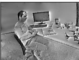
CMax-anchor
