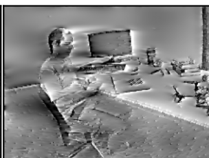
CMax-anchor
