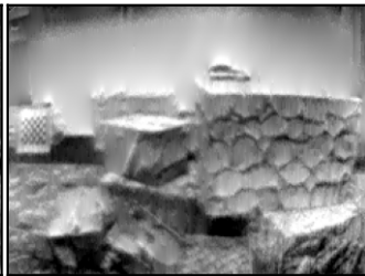
|r| = 0.84
