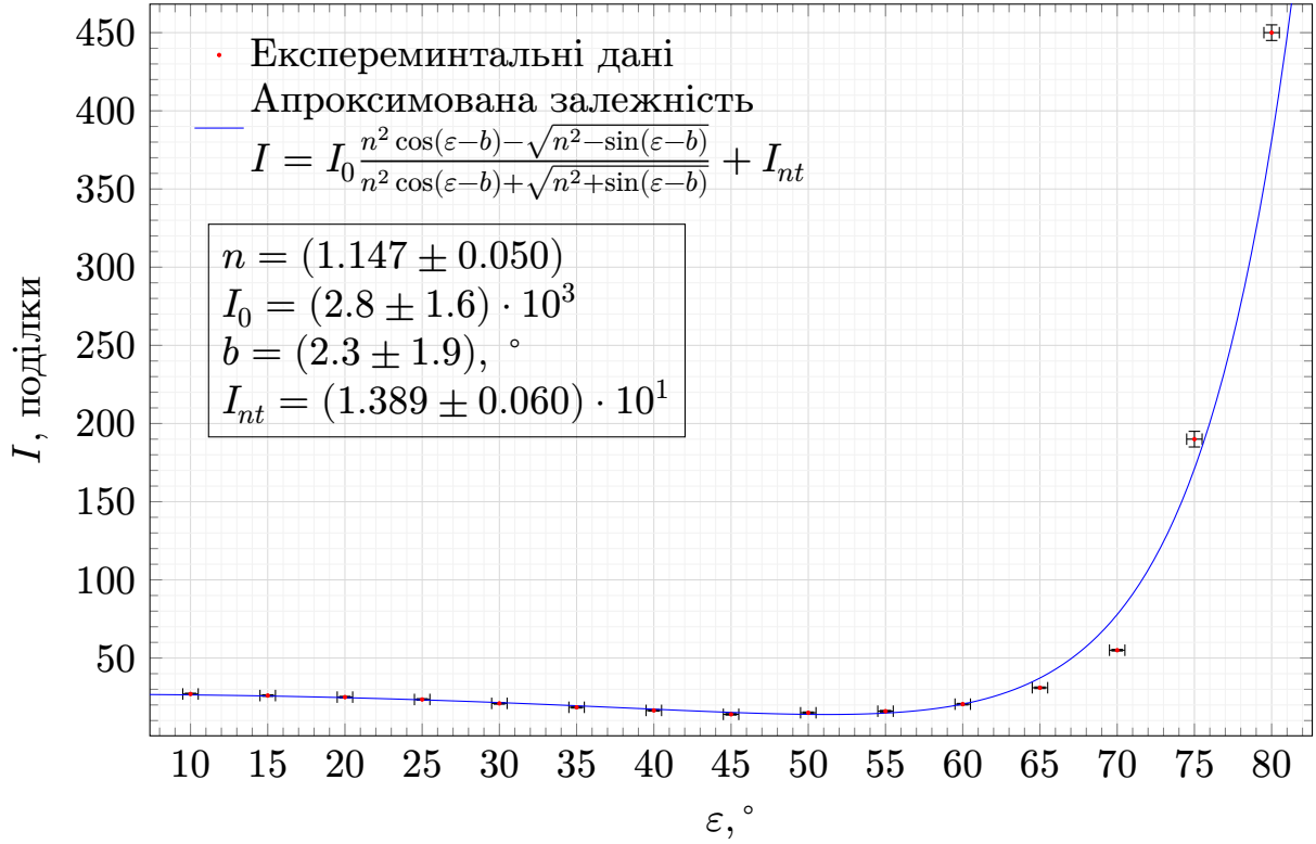
Рис. 5: залежність I(\alpha) . Знаходження n чорного дзеркала
