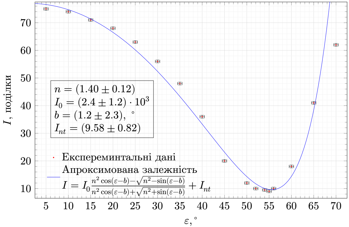
Рис. 6: залежність I(\alpha) . Знаходження n стопи пластин
