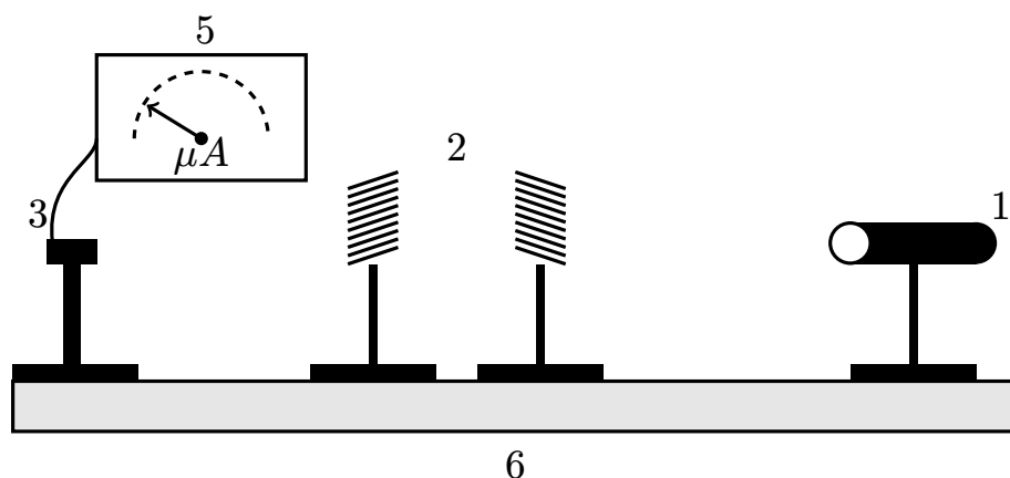
Рис. 1: Експериментальна установка до 1 досліду
