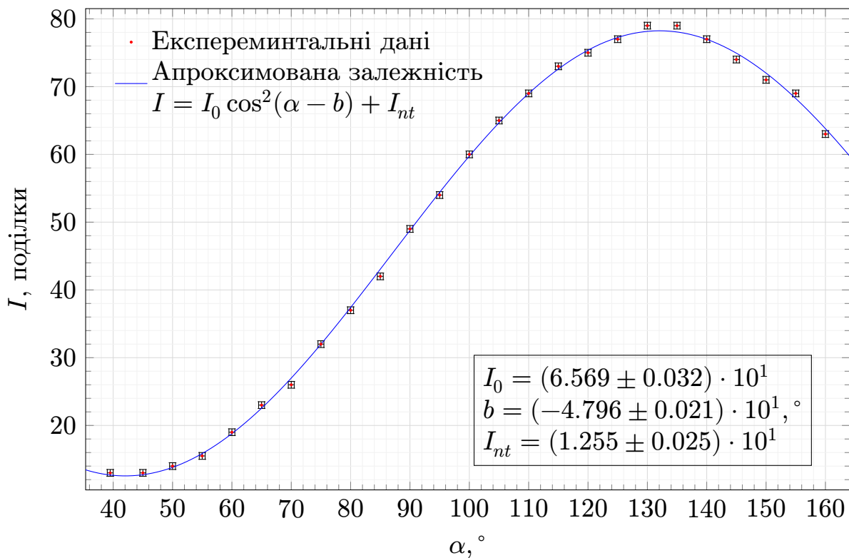
Рис. 2: Залежність I(\alpha) встановлена під час незавершеного експерименту з поляроїдами
