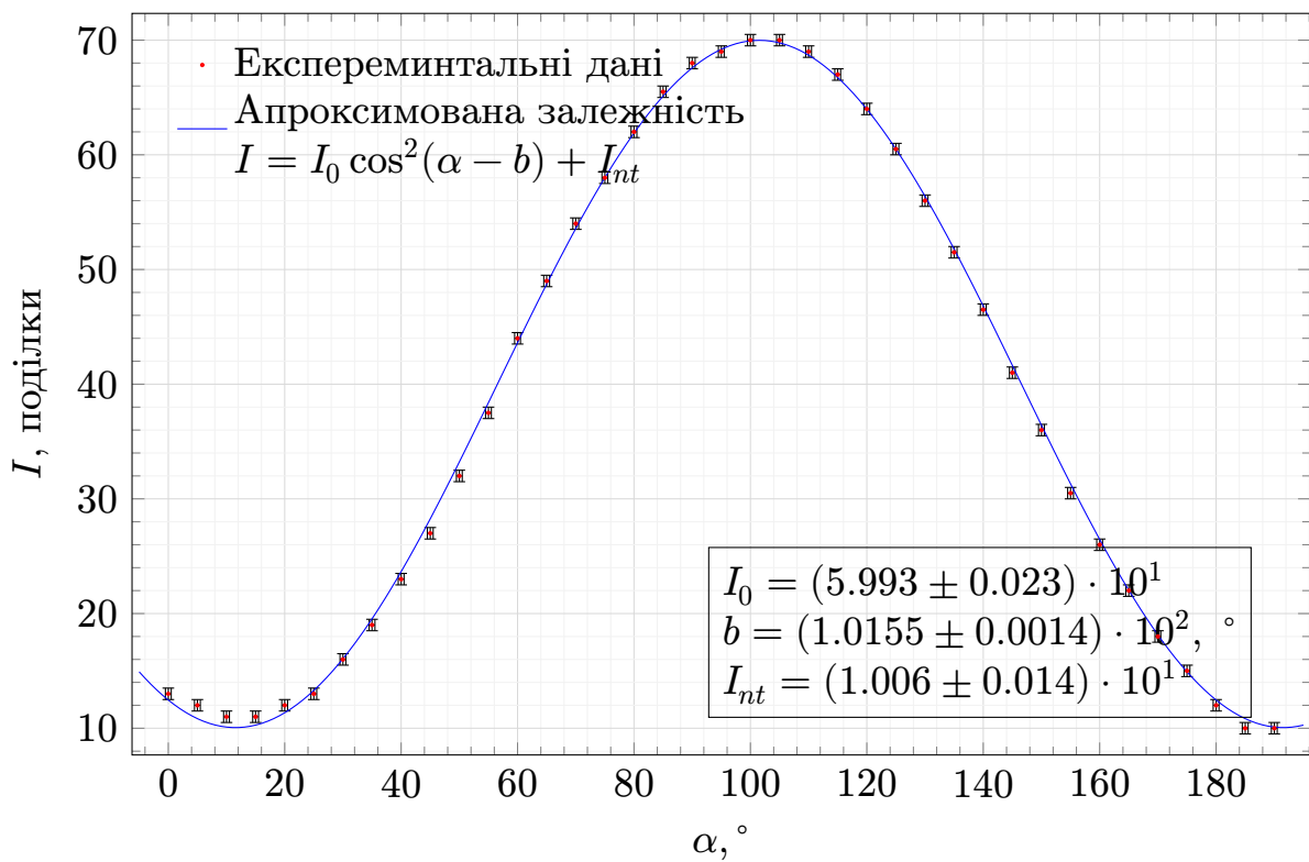
Рис. 3: залежність I(\alpha) для повноцінного експерименту з поляроїдами
