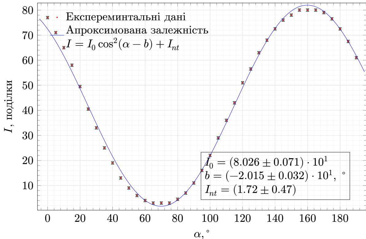
Рис. 4: залежність I(\alpha) для експерименту з призмою Ніколя
