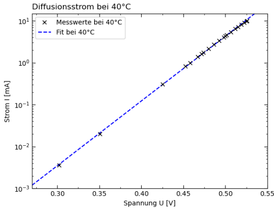
Abb. 5: Halblogarithmische Auftragung des Diffusionsstroms I_D gegen die angelegte Spannung U für T = 40^\circ\text{C}
