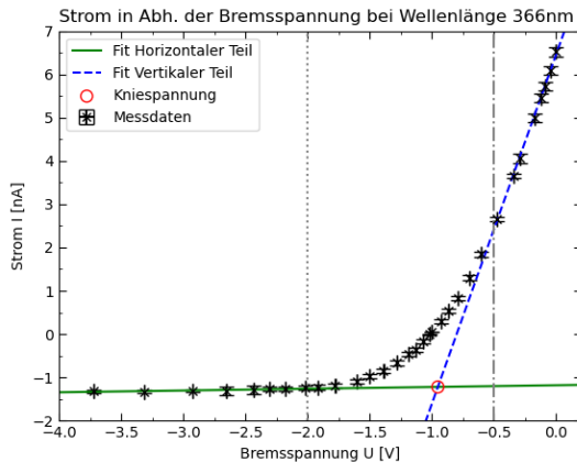
Abb. 1: Bremsspannung für \lambda = 366 \text{ nm}
