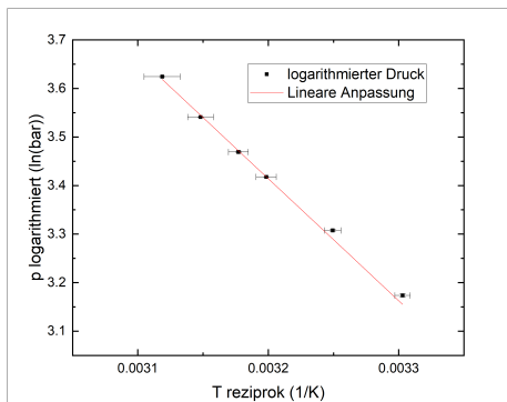
Abb. 3: Auftragung der logarithmierten Dampfdruckkurve von SF_6
