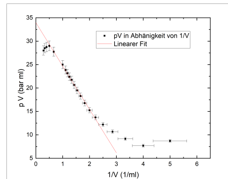
Abb. 4: Bestimmung der Stoffmenge von SF_6 durch lineare Anpassung im thermodynamischen Limes
