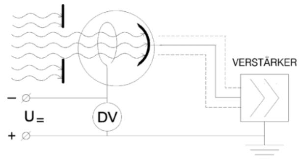
Abb. 1: Schematischer Versuchsaufbau zur Bestimmung des Planckschen Wirkungsquantums mit einer Quecksilberhochdrucklampe [1]
