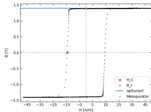
Abb. 7: Aufgenommene Hysteresekurve der Nickel-Eisen-Legierung PERMENORM 5000 Z.
