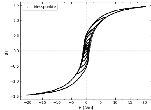
Abb. 6: Entmagnetisierung eines Eisenkerns durch sukzessive Verringerung des maximalen Magnetfeldes nach jeder Umpolung.
