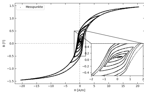
Abb. 7: Entmagnetisierung eines Eisenkerns durch sukzessive Verringerung des maximalen Magnetfeldes nach jeder Umpolung.
