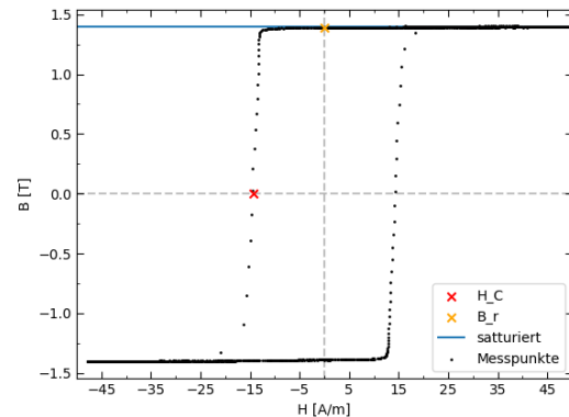
Abb. 8: Aufgenommene Hysteresekurve der Nickel-Eisen-Legierung PERMENORM 5000 Z.
