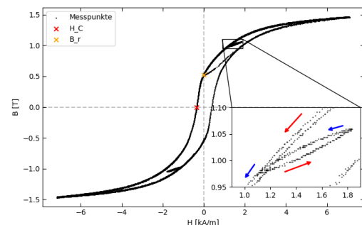
Abb. 6: Untersuchung der Irreversibilität der Magnetisierung eines Eisenkerns durch Richtungsänderung.
