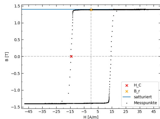
Abb. 5: Aufgenommene Hysteresekurve der Nickel-Eisen-Legierung PERMENORM 5000 Z.
