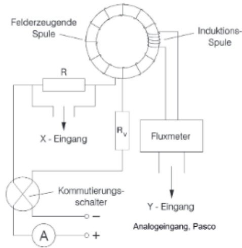
Abb. 1: Versuchsaufbau zur Messung der Hysteresekurven [?].
