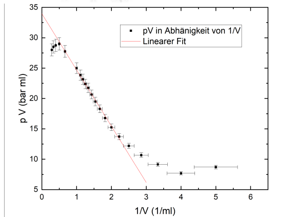
Abb. 5: Bestimmung der Stoffmenge von SF_6 durch lineare Anpassung im thermodynamischen Limes
