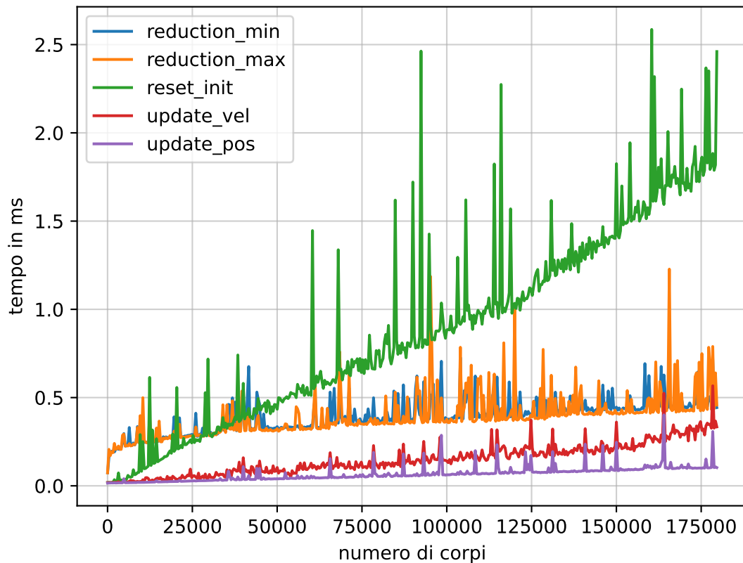
tempo di dei vari kernel Barnes-Hut (10 iterazioni, \theta = 0.1 ), pt.1
