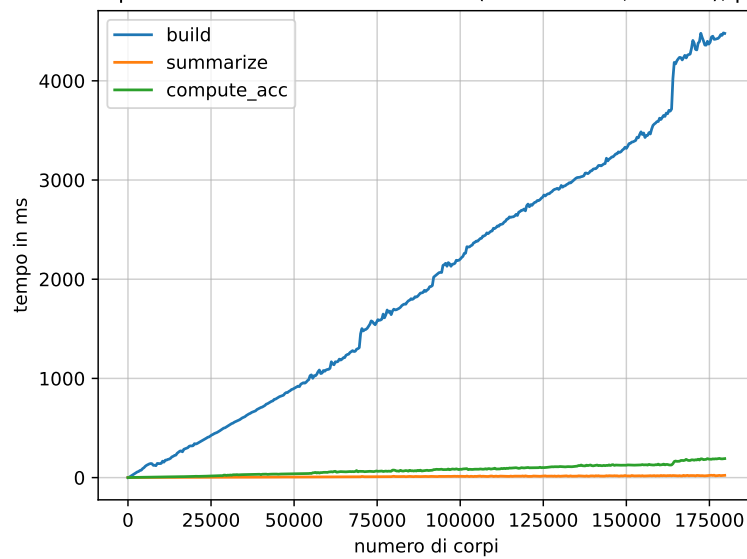
tempo di dei vari kernel Barnes-Hut (10 iterazioni, \theta = 0.5 ), pt.2
