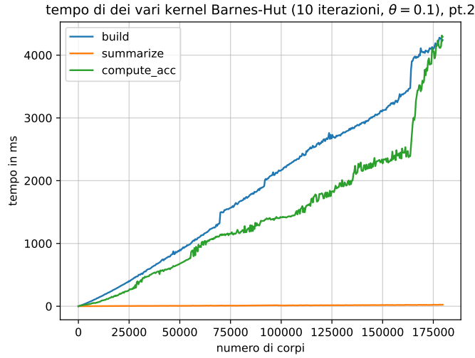
Immagine 10: Plot dei tempi dei kernel di costruzione (seriale) dell'albero, propagazione di masse e centri di massa e calcolo dell'accelerazione in funzione del numero di corpi, con \theta = 0.1
