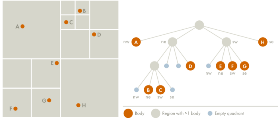
Immagine 7: Bounding box e quad-tree nell'algoritmo Barnes-Hut, immagine tratta da https://arborjs.org/docs/barnes-hut
