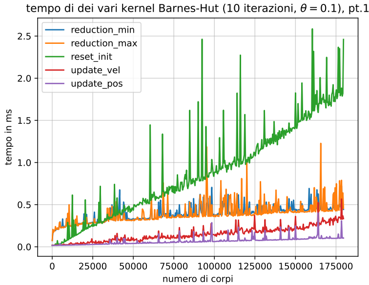
Immagine 9: Tempo dei kernel di Barnes-Hut per la riduzione (minimo e massimo della bounding-box), reset e inizializzazione dell'albero, aggiornamento della velocità e della posizione.
