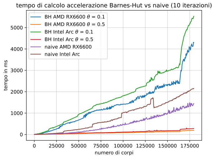
Immagine 12: Plot dei tempi dei kernel di calcolo dell'accelerazione nell'approccio naive e nell'approccio Barnes-Hut con \theta = 0.1 e \theta = 0.5 .
