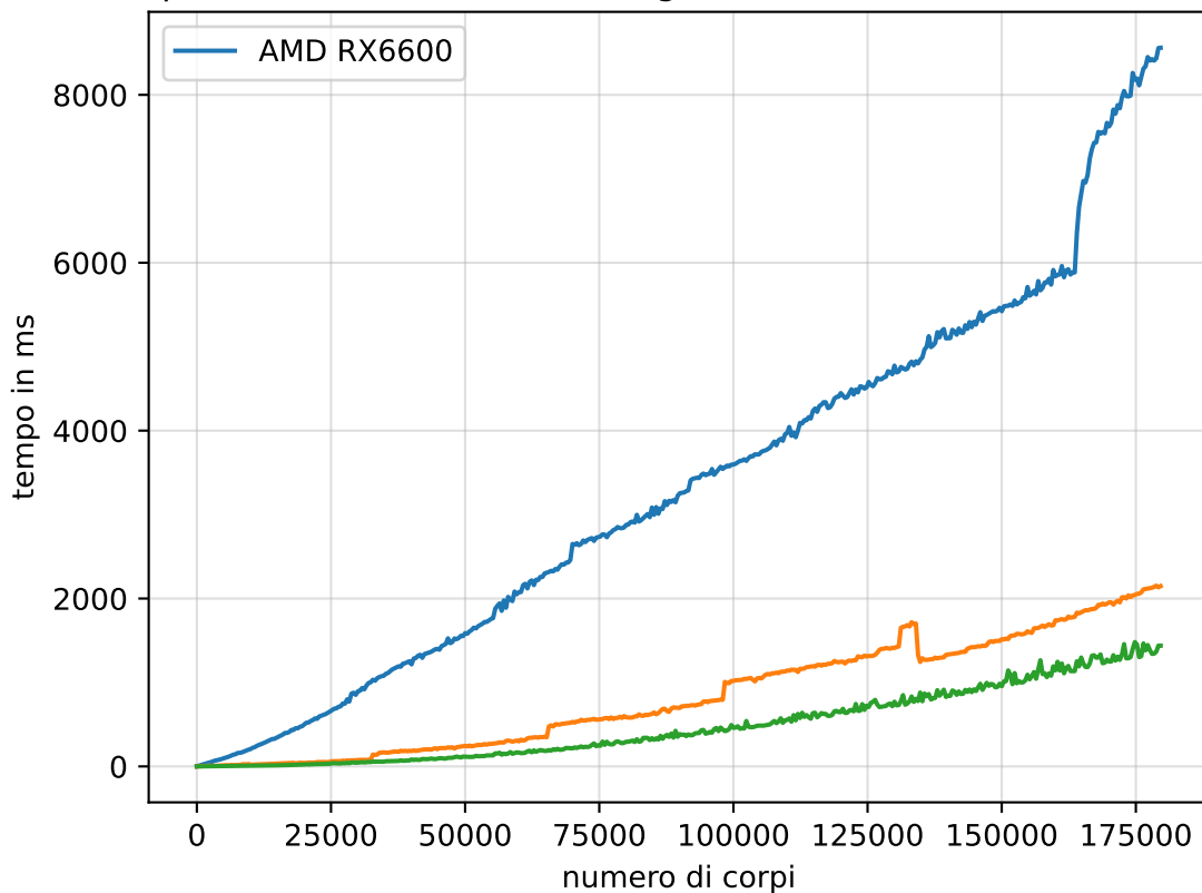
tempo dei kernel di riduzione algoritmo Barnes-Hut (10 iterazioni)
