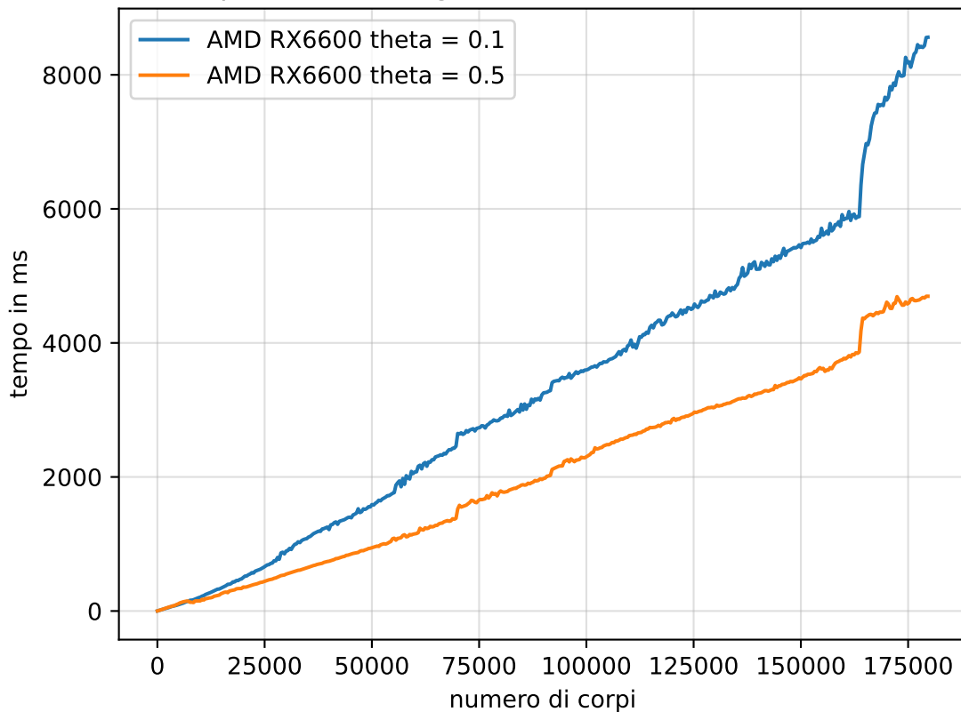
tempo di calcolo algoritmo Barnes-Hut (10 iterazioni)
