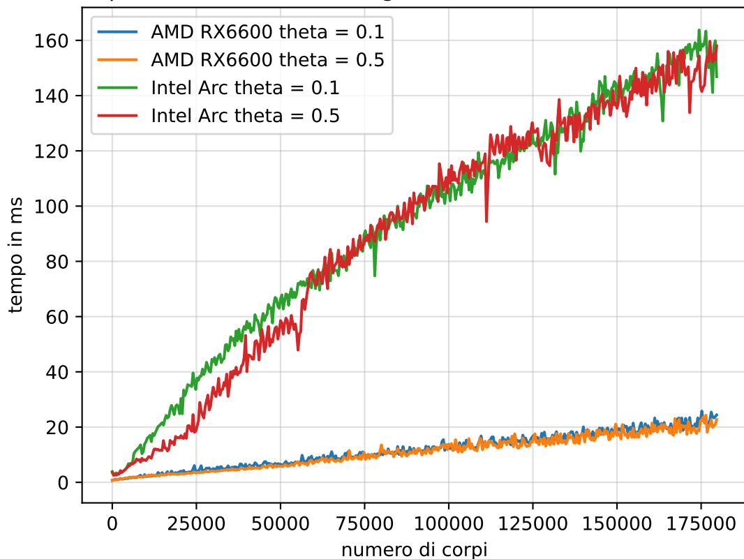
tempo di summarize tree, algoritmo Barnes-Hut (10 iterazioni)
