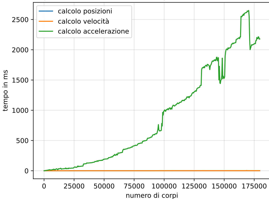
tempo di calcolo dei kernel nell'algorithm naive (10 iterazioni)
