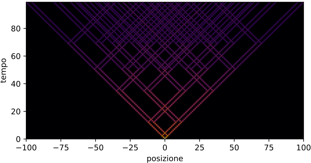
Passeggiata aleatoria quantistica, canale H, p=0.95
