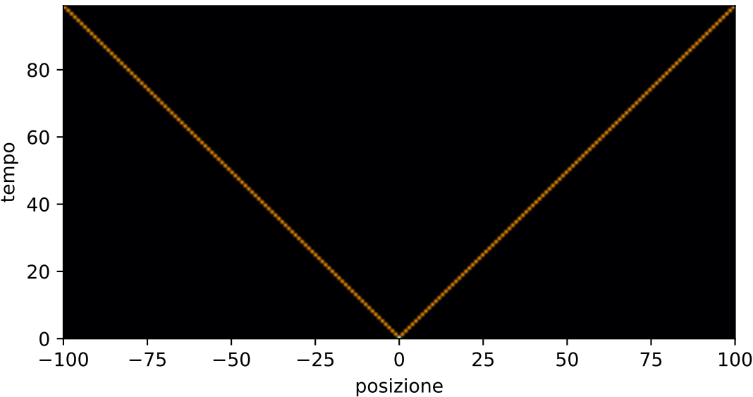
Passeggiata aleatoria quantistica, canale H, p=1
