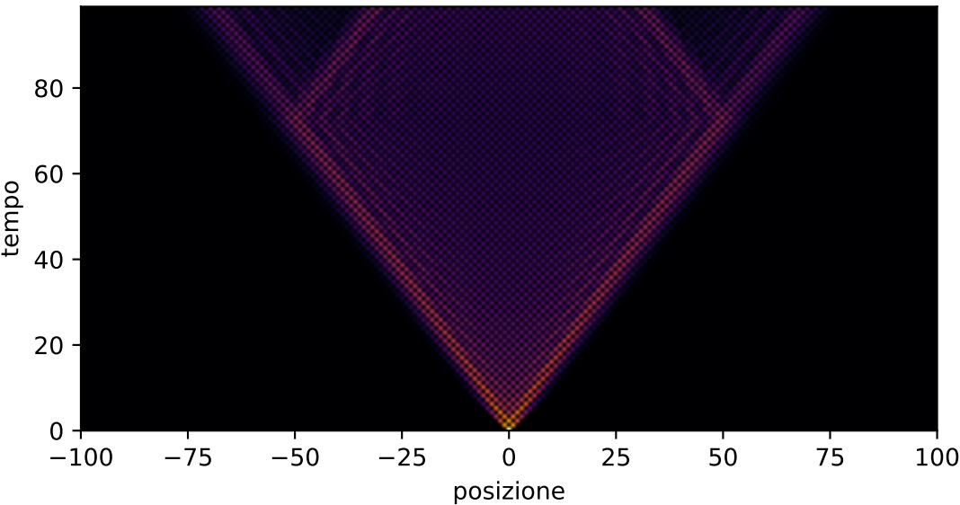
Passeggiata aleatoria quantistica, canale X, p=0.01
