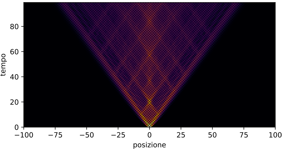
Passaggiata aleatoria quantistica, canale meas, p=0.05
