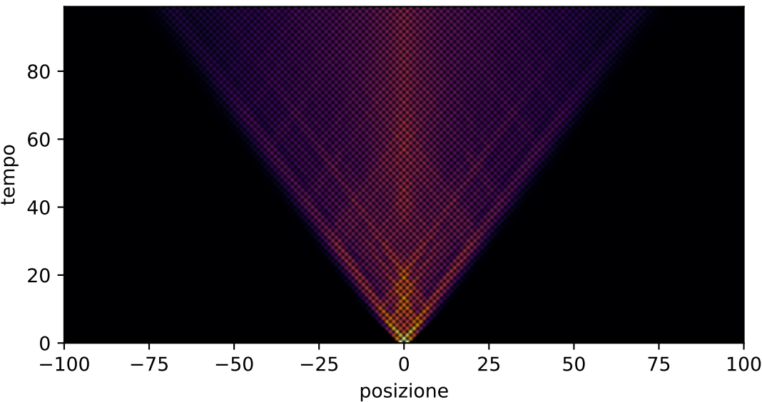
Passaggiata aleatoria quantistica, canale meas, p=0.08
