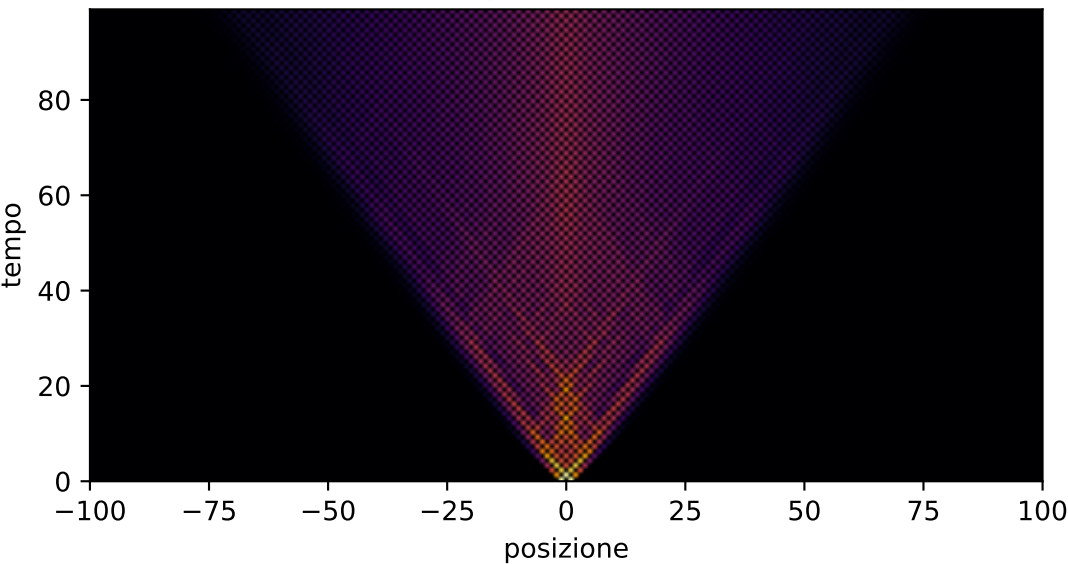
Passaggiata aleatoria quantistica, canale meas, p=0.13
