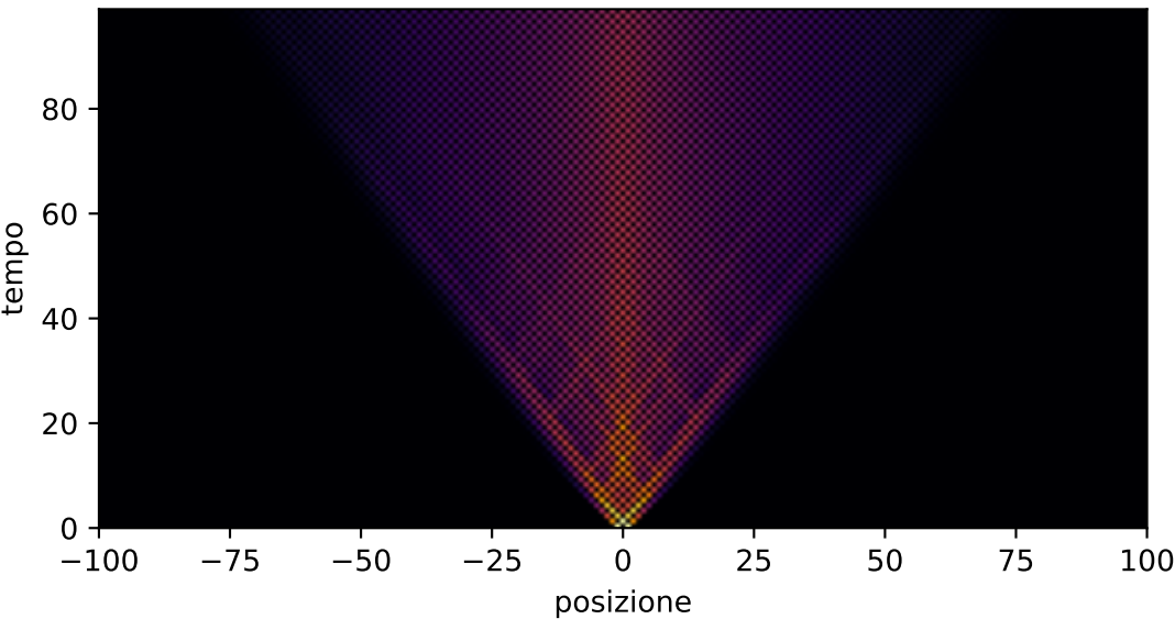
Passeggiata aleatoria quantistica, canale meas, p=0.15
