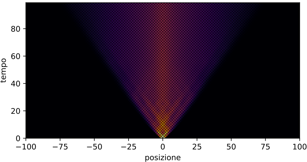
Passeggiata aleatoria quantistica, canale meas, p=0.18
