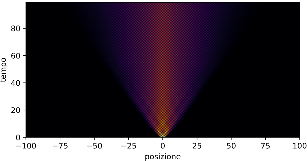
Passeggiata aleatoria quantistica, canale meas, p=0.21
