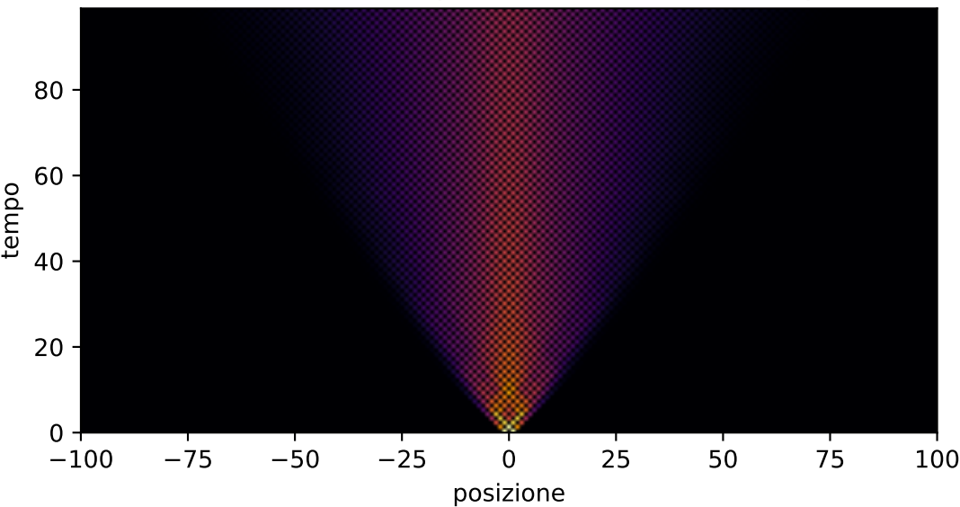
Passaggiata aleatoria quantistica, canale meas, p=0.26
