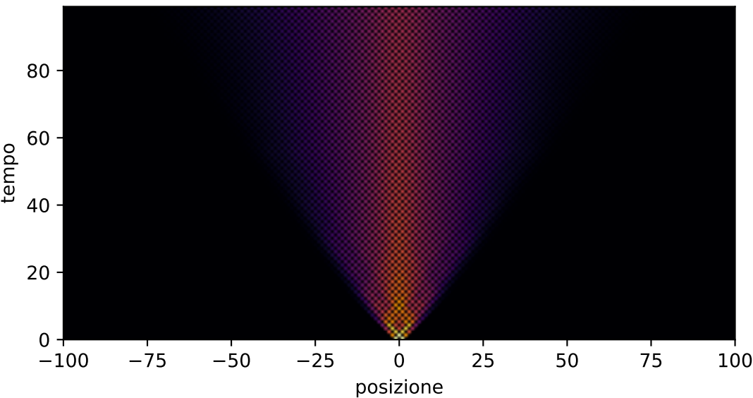
Passaggiata aleatoria quantistica, canale meas, p=0.28
