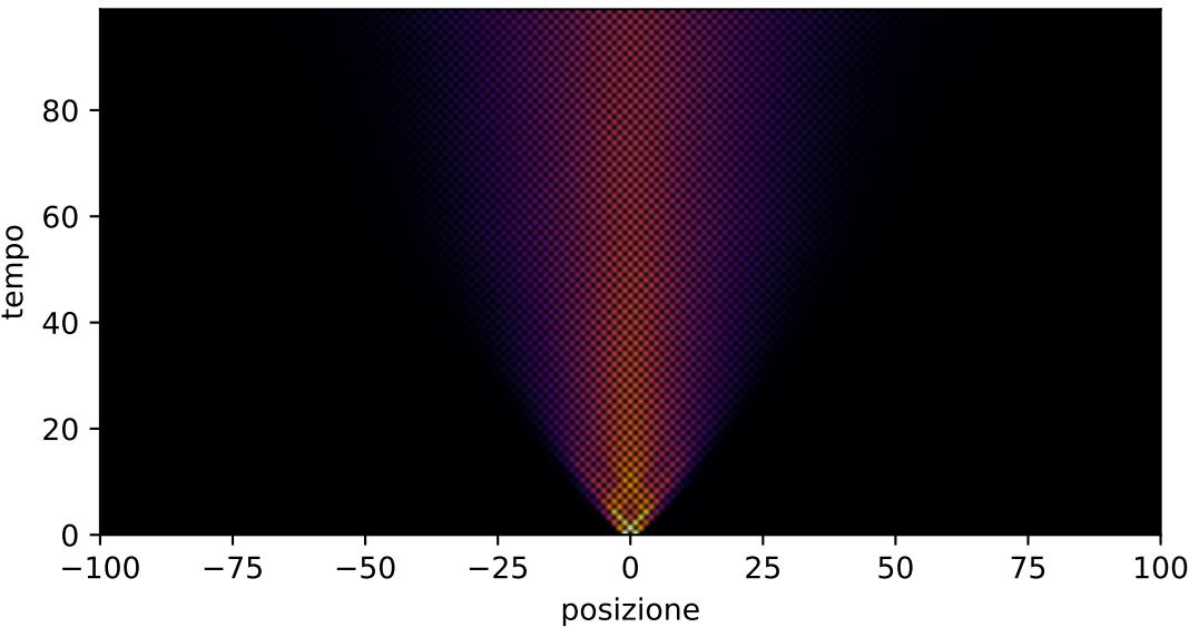
Passaggiata aleatoria quantistica, canale meas, p=0.41
