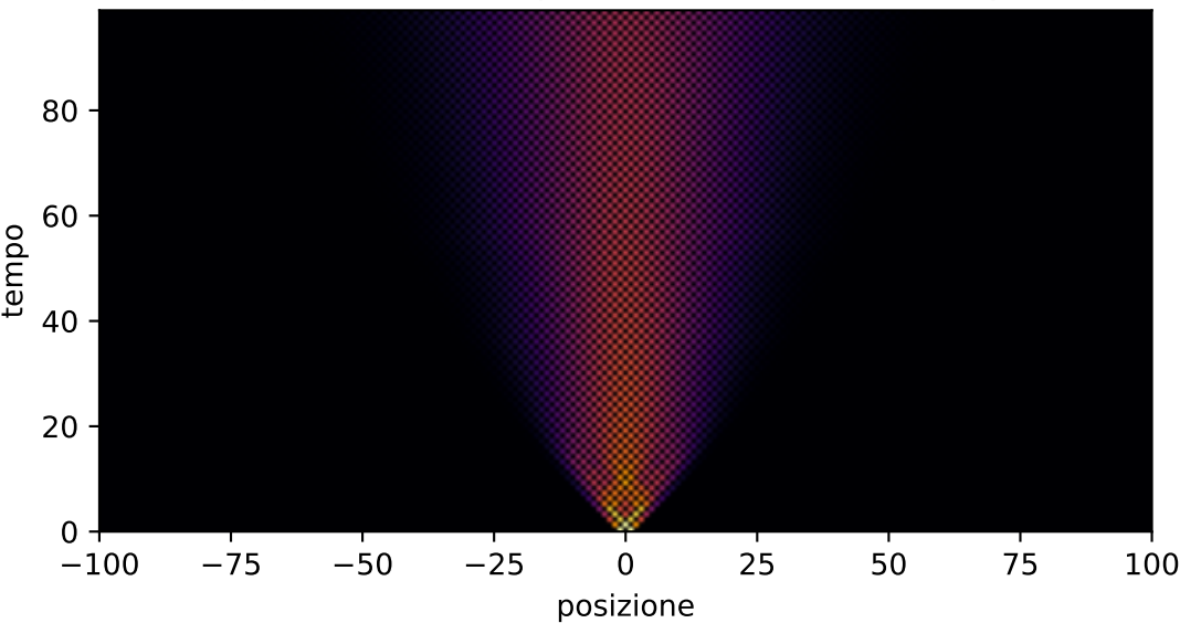
Passeggiata aleatoria quantistica, canale meas, p=0.54
