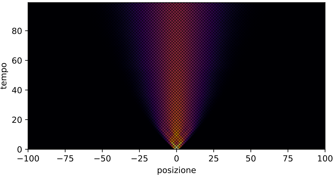
Passeggiata aleatoria quantistica, canale meas, p=0.56
